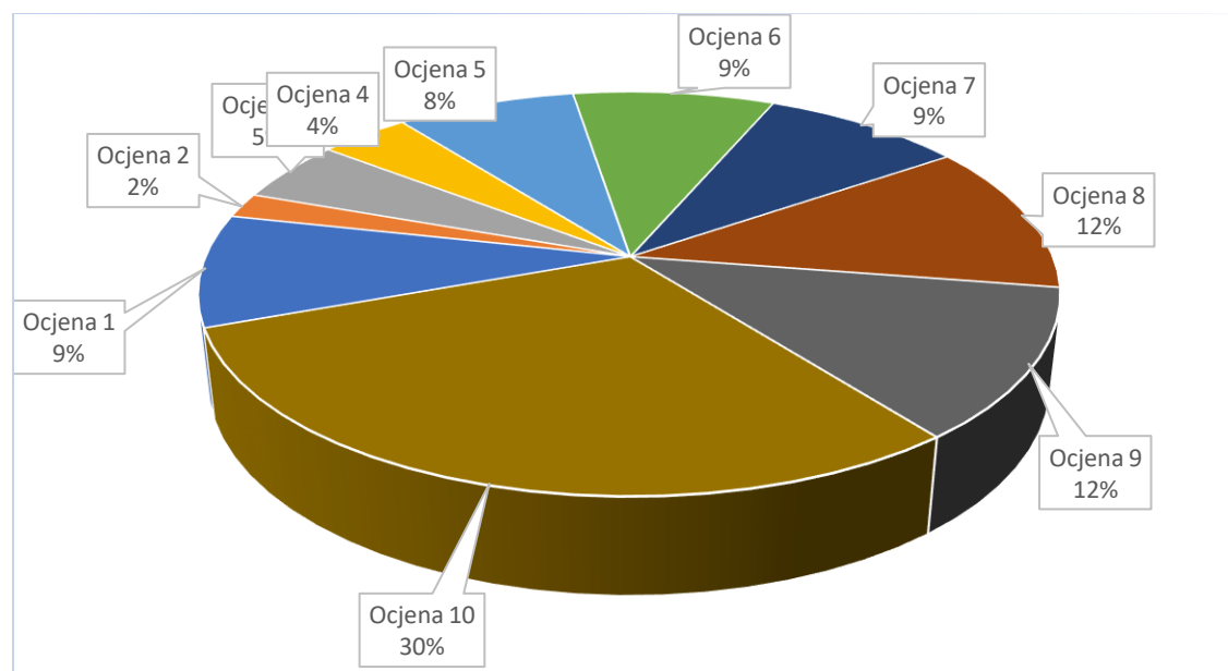
Grafik 1: Važnost osnivanja omladinskog servisa, kluba ili centra: Ocjene mladih na skali od 1 do 10
